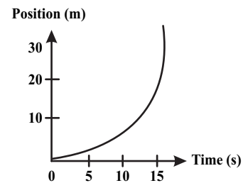
Figure 1.12 Non linear graph
