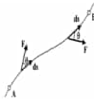
Fig: 5.5 Variable force
