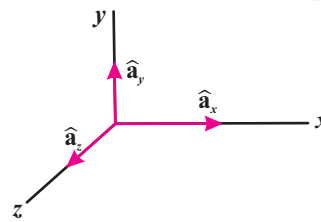
Fig: 2.6 Cartesian coordinates
