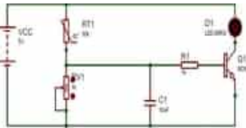
Fig: 10.11 Thermostat
