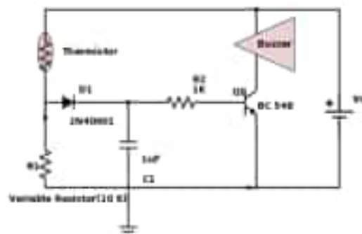
Fig: 10.10 Fire Alarm
