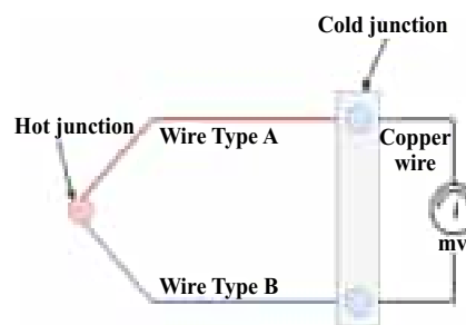
Fig:10.8 Thermocouple
